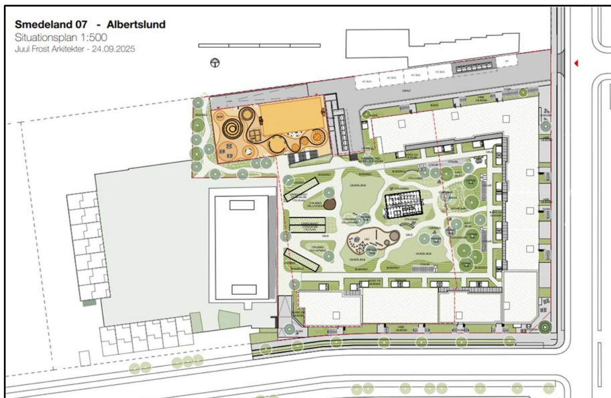
Figur 1. Foreløbig situationsplan for projekteret indretning af Smedeland 7.
