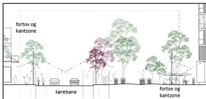
Figur 5 Smedeland, tværprofil fra Masterplan for Hersted Industripark
