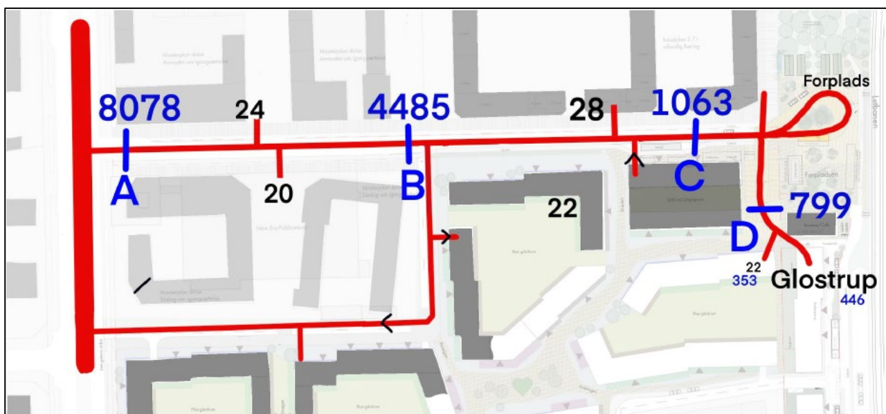
Figur 10: Beregnede trafikmængder på Hersted Stationsvej (Sweco 2024). Beregningen omfatter ture til/fra boliger, som forventes at benytte Hersted Stationsvej, ture til/fra planlagte butikker langs Hersted Stationsvej og ture til/fra busstop og afsætningsplads ved letbanestationen.
