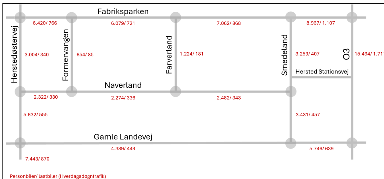
Figur 11: Basisscenariet viser beregnede trafikmængder, der i så vidt omfang som muligt svarer til den faktiske trafik målt ved tællinger i 2025 og er fremskrevet med 0,2 procent i henhold til Vejdirektoratets forventede årlige vækst i trafikarbejdet.
