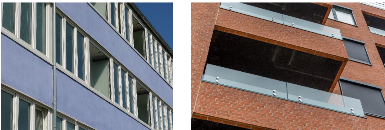
Figur 36. I ejendommen til venstre blev altanerne forsynet med en forsatsrude, der kan skydes til siden. Når ruden er lukket, fungerer den sammen med altanrummet som en meget effektiv støjdæmpning. Til højre er vist åbne altaner med en glasafskærmning, der begrænser støjen. Der er desuden et lydabsorberende akustikloft, som dæmper støjen i altanrummet.
