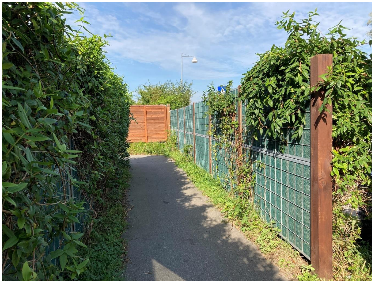
Figur 27. Eksempel på støjskærm ved et boligområde. De grønne akustiske elementer i skærmen består af lydabsorberende mineraluld.
