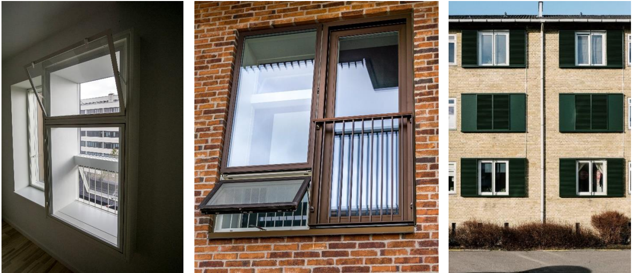
Figur 35. Støjdæmpende multifunktionsvindue (billedet til venstre og billedet i midten). Støjen dæmpes på vejen gennem åbningen for neden (udendørs) til åbningen for oven (indendørs). Til højre er vist en lydskodde, som er monteret foran et eksisterende vindue. Den dæmper støjen, men giver også adgang for frisk luft. Den kan desuden mørkelægge et rum, hvis det ønskes.
