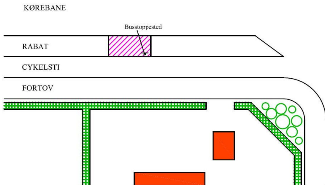
Figur 12, Busstoppested med særskilt busperron mellem cykelsti og kørebane.
