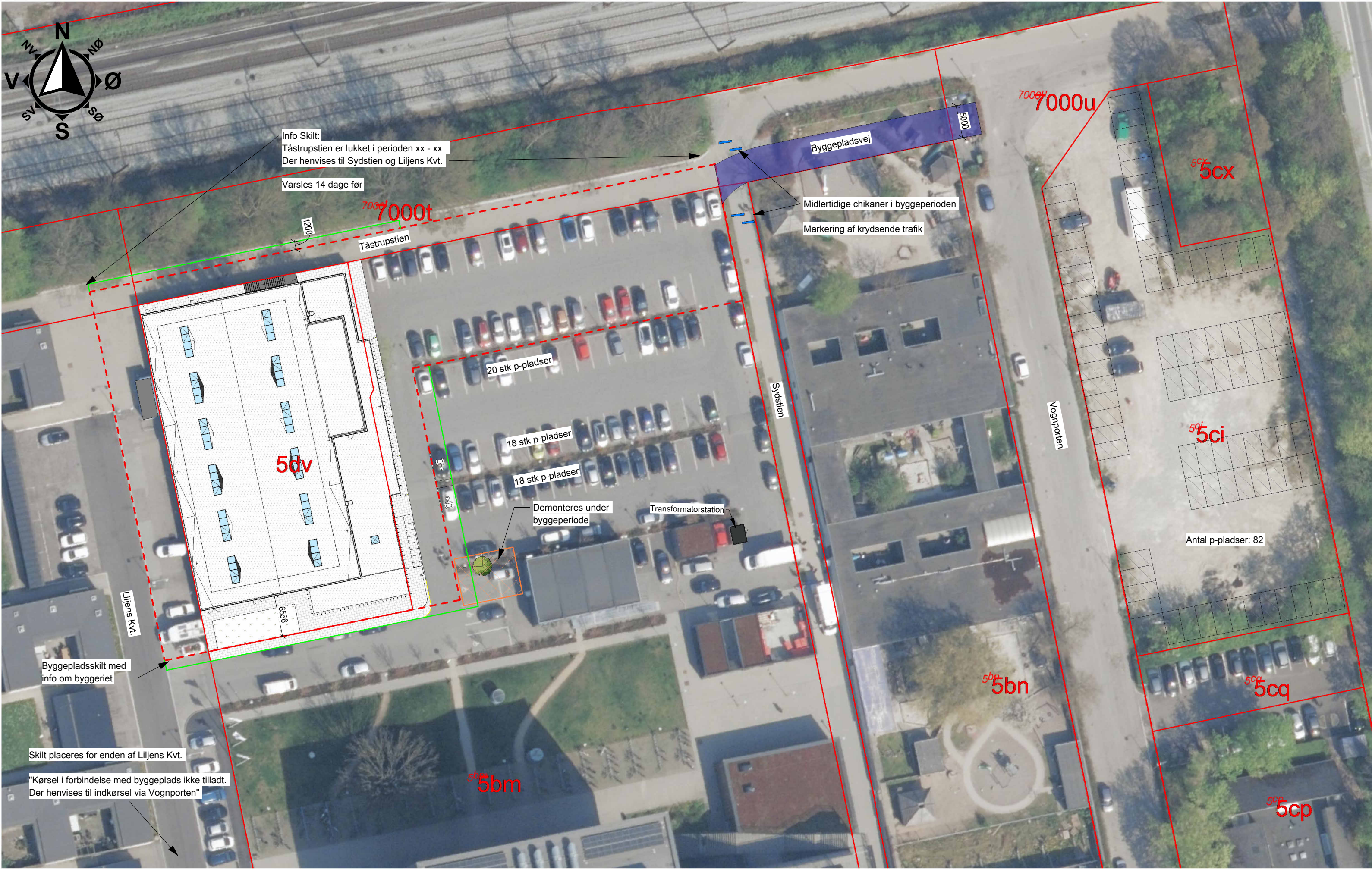
Byggeplads plan, 1 : 500
