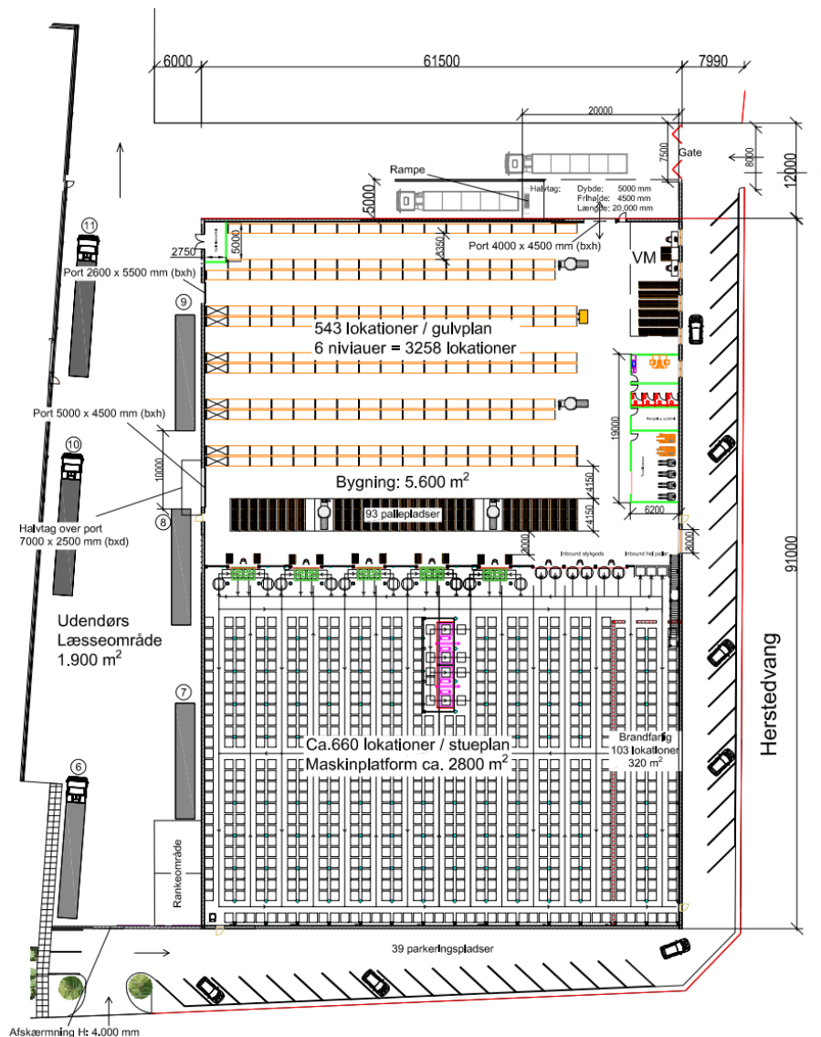
Figur 1: Situationsplan for projektområdet, fremtidige forhold
