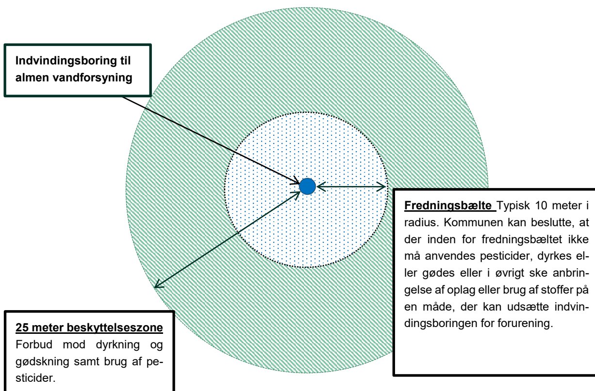
Figur 2.1: Konceptuel figur af 25 meter beskyttelseszone og fredningsbælte udlagt i forbindelse med en indvindingsboring der indvinder vand til almen vandforsyning.
