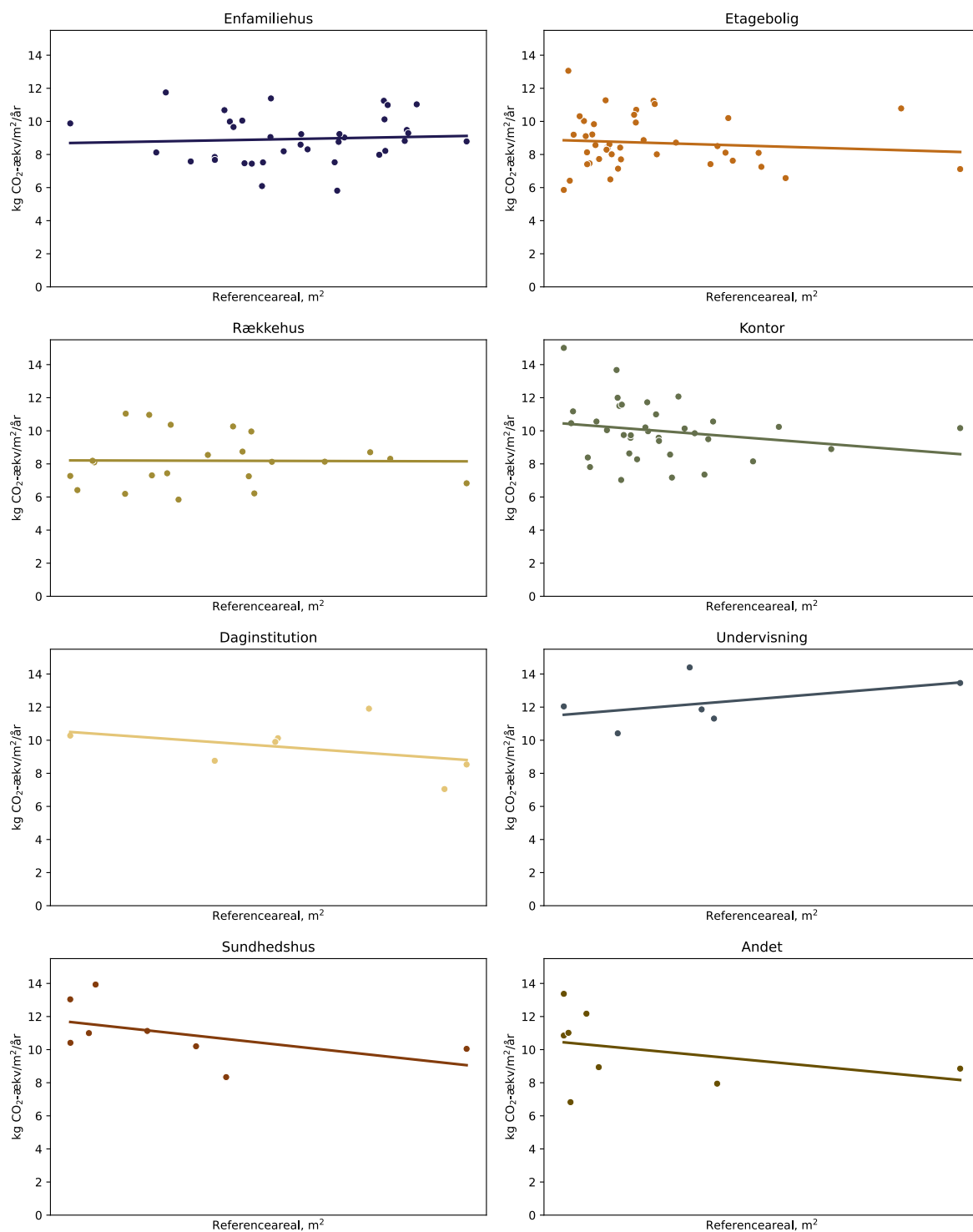
Figur 42. Tendenslinje for samtlige bygningsanvendelser for at vise en eventuel sammenhæng mellem referenceareal i m² og klimapåvirkningen.
