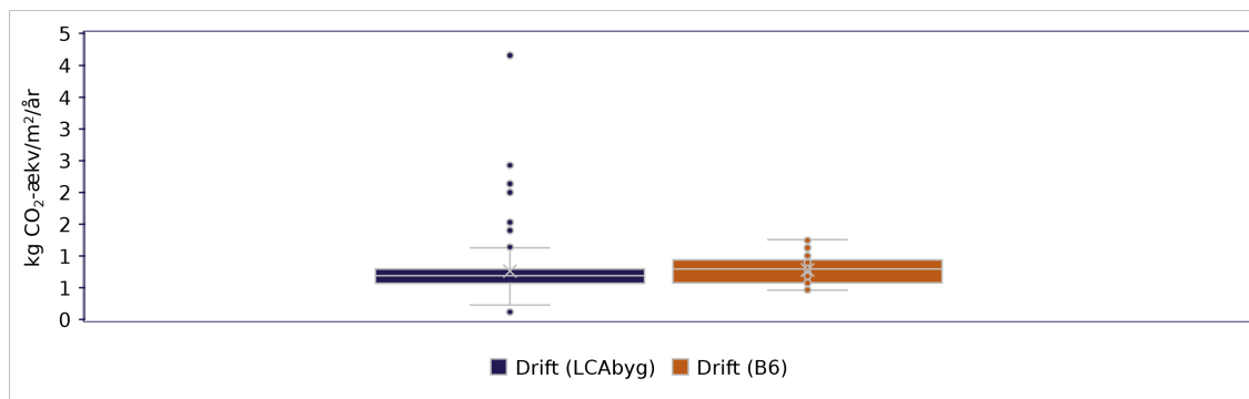
Figur 35. Boxplot over klimapåvirkning fra drift indtastet i LCAbyg og det normaliserede forbrug (maksimale forbrugt iht. energirammen).
