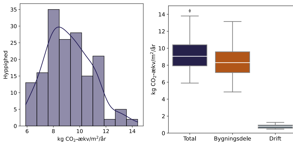
Figur 19. Histogram over samlede klimapåvirkning (A1-3, B4, B6, C3-4) og boksplot over klimapåvirkningen for henholdsvis total (A1-3, B4, B6, C3-4), bygningsdele (A1-3, B4, C3-4) og drift (B6). Klimapåvirkningen er opgjort i kg CO 2 -ækv/m 2 /år med betragtningsperiode på 50 år.
