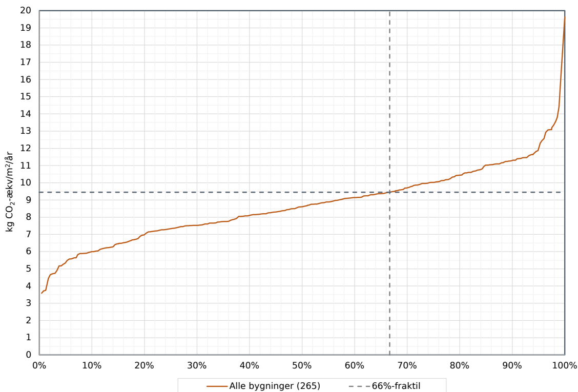
Figur 48. Fordelingskurve for den vægtede klimapåvirkning over 265 case-bygninger med markering af 66%-fraktilen, der viser, hvor grænseværdien ligger for at fastlægge 1/3-ambitionsniveauet. Klimapåvirkningen er opgjort i kg CO 2 -ækv/m 2 /år med betragtningsperiode på 50 år.
