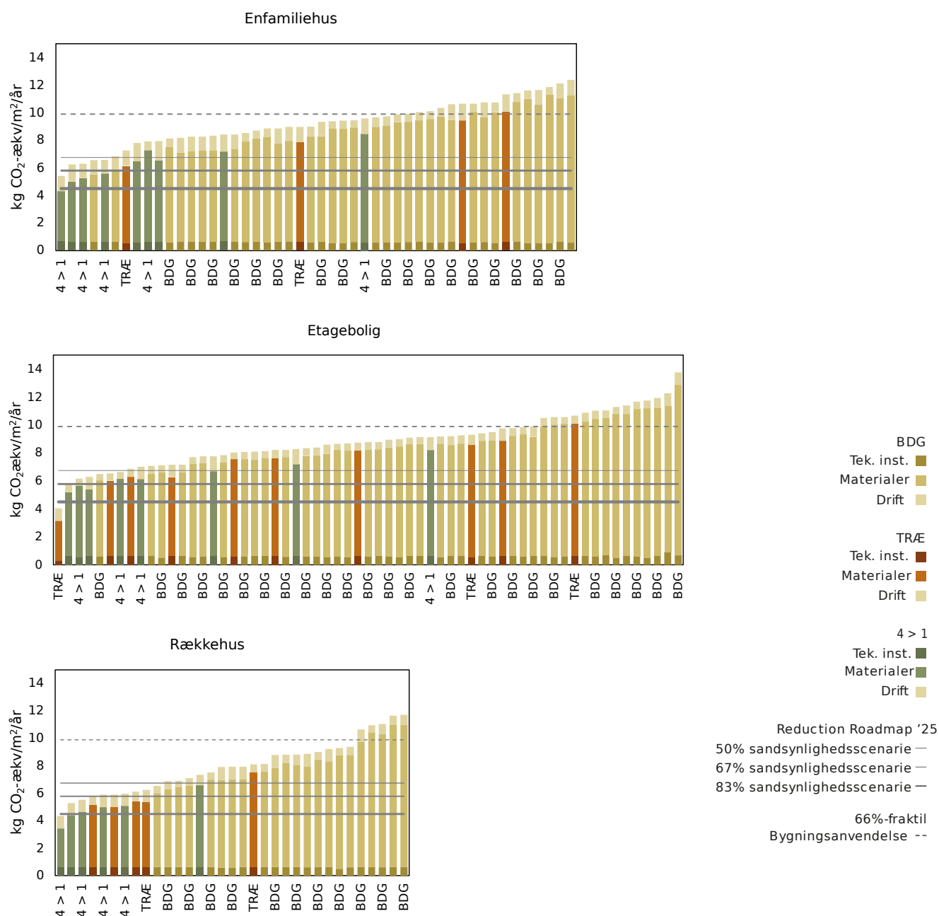
Figur 47. Klimapåvirkning opgjort i kg CO 2 -ækv/m 2 /år over en betragtningsperiode på 50 år fordelt i bolig kategorier inkluderet cases fra BUILD rapport 2023:10 Klimapåvirkning fra: 45 Træbyggerier og BUILD rapport 2023:12 Boligbyggeri fra 4 til 1 planet: 25 Best Practice Cases .
