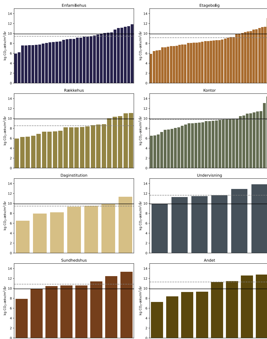
Figur 24. Søjlediagrammer over ikke-vægtede klimapåvirkninger (A1-3, B4, B6, C3-4) for de 8 kategorier af bygningsanvendelser. Vandrette linjer indikerer 66%-fraktalen for den specifikke bygningsanvendelse (stiplet, grå) og den sorte viser den samlede 66%-fraktal.
