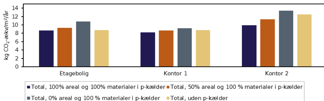
Figur 40. P-kælders betydning for bygningens klimapåvirkningen ved forskellige arealer
