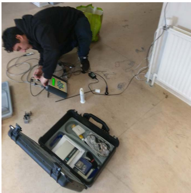
En praktisk test af en typisk radiator. Der bliver logget maksimalt flow gennem radiatoren, samt temperatur på både fremløb og retur.
